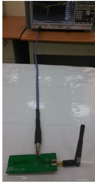
Antenna R/A
