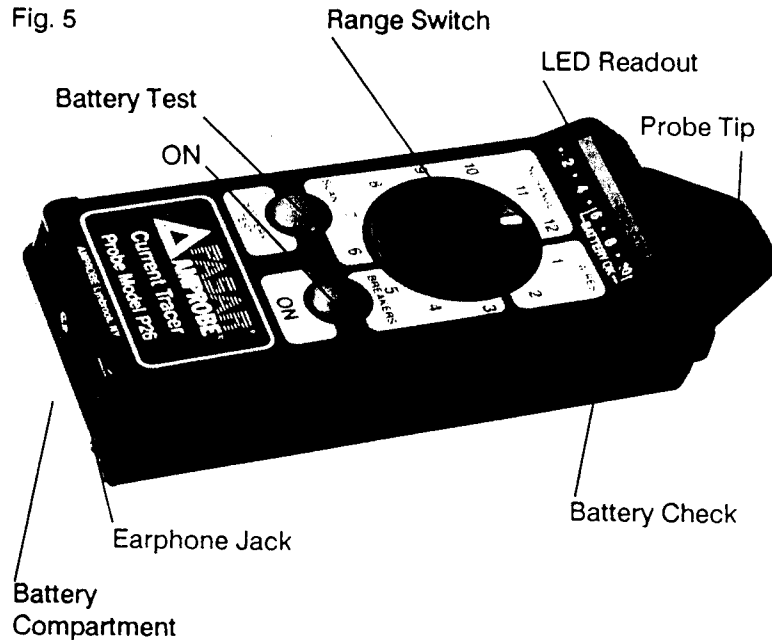
P26 Probe
